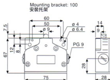
Mounting bracket: 100 安裝托架
