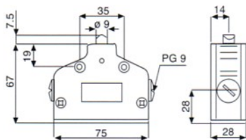
Mounting bracket: 100 安裝托架
