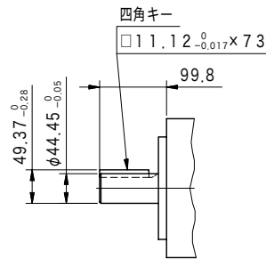
軸端形状
