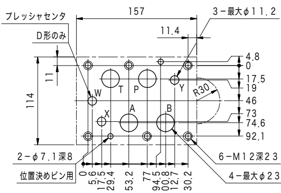
取付面寸法 (ISO 4401-AE-08-4-A 準拠)
