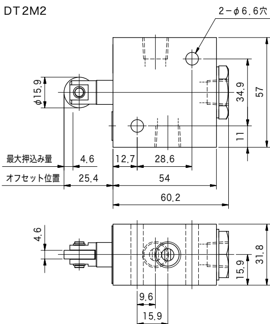
DT2M2
