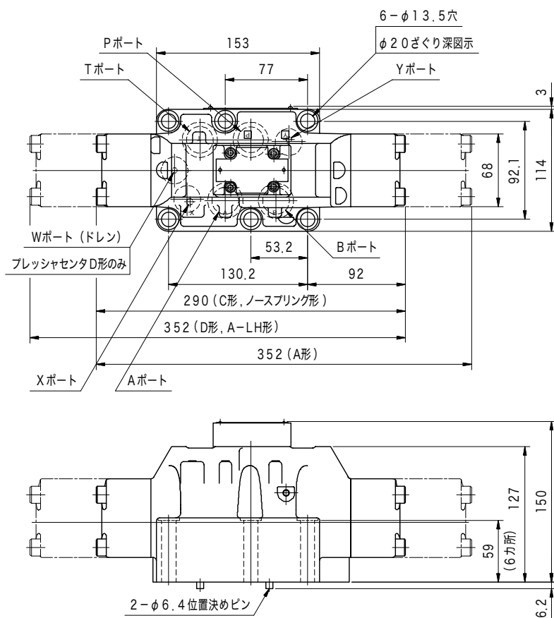
DG3V-H8
