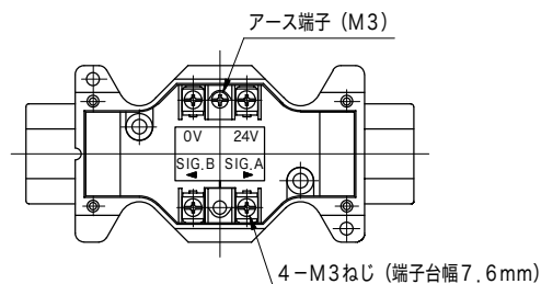
PS2形
