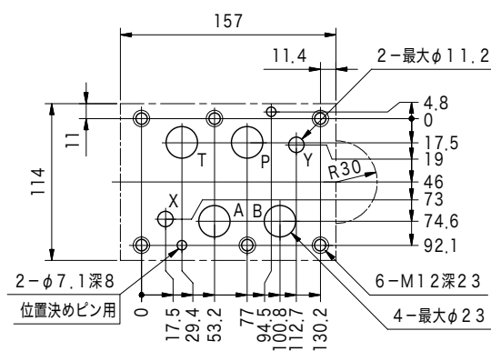
●取付面寸法 (ISO 4401-AE-08-4-A準拠)
