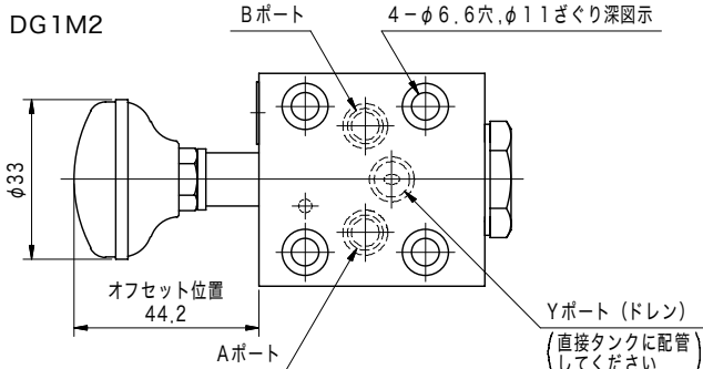
取付面寸法
