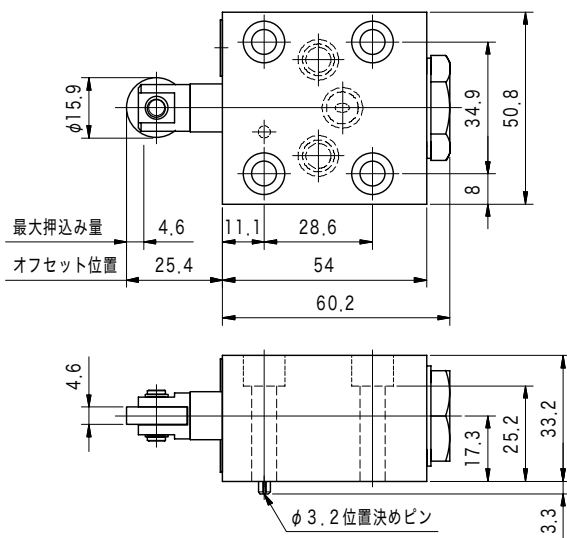
DG2M2
