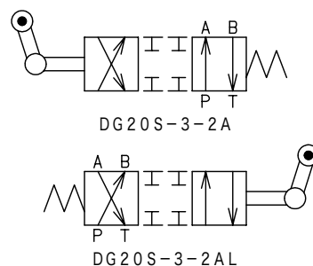
油圧図記号
