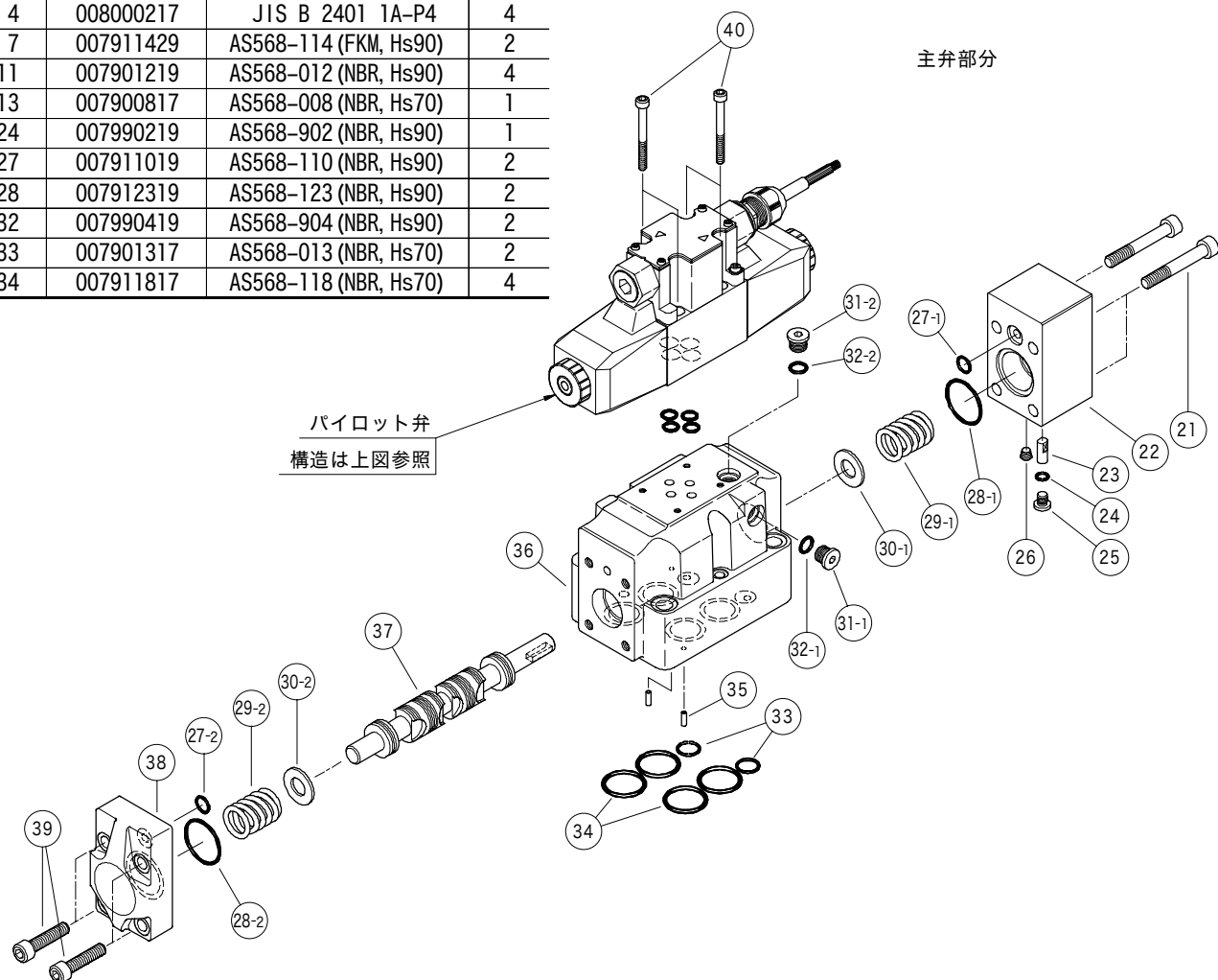
Oリング COM-7
