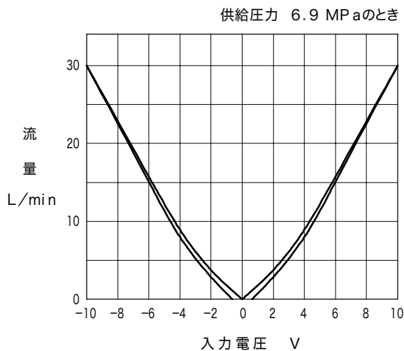
入力電圧－流量特性
