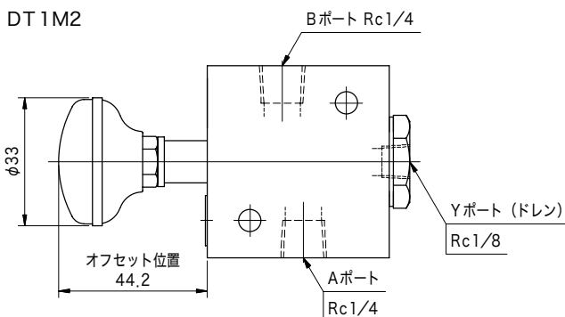
DT1M2
