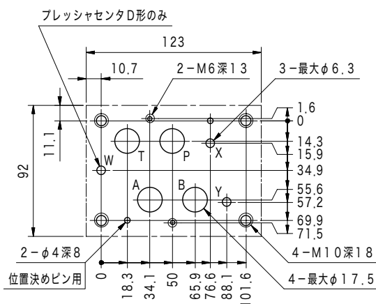
取付面寸法 (ISO 4401-AD-07-4-A 準拠)
