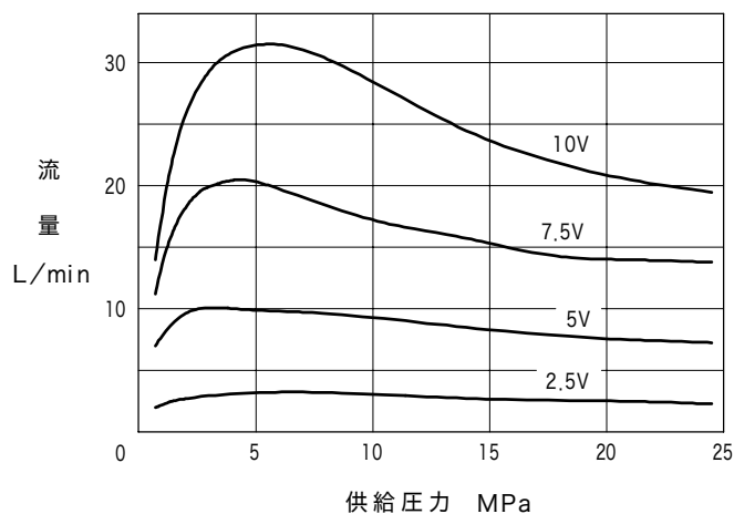
供給圧力－流量特性
